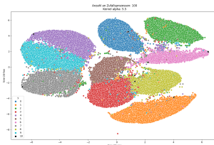
(e) 100 Zufallsprozesse, \alpha = 5.5
