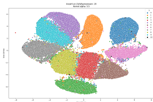
(d) 20 Zufallsprozesse, \alpha = 5.5
