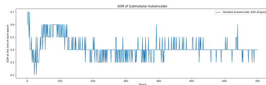
(h) SDM-Accuracies des DSA mit \alpha = 3.1 , \lambda = 0.1
