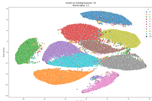
(a) 20 Zufallsprozesse, \alpha = 3.1
