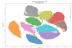
(l) 500 Zufallsprozesse, \alpha = 10.0
