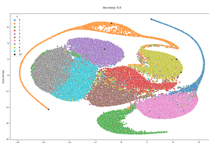
(k) Nach Epoche 300 \alpha = 10.0 \lambda = 0.1
