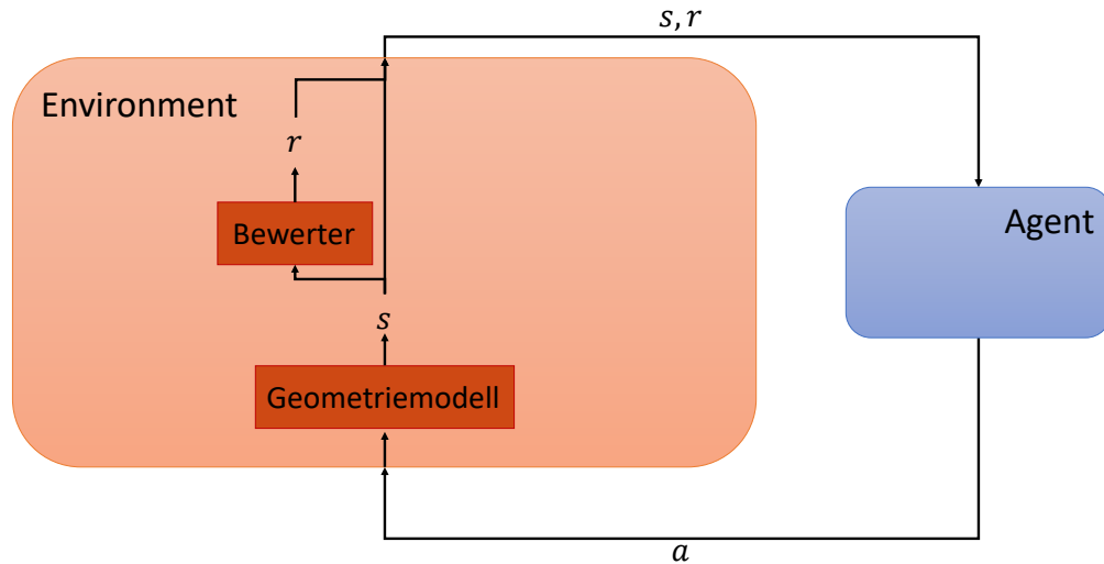
Abbildung 3.3: Environment-Architektur: Das Environment besteht aus zwei Komponenten: dem Geometriemodell und dem Bewerter. Während das Geometriemodell die neue Beladung berechnet, bewertet der Bewerter diese. Zusammen ergibt dies das Feedback des Environments.
