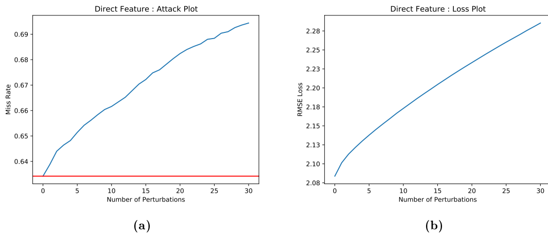
Abbildung C.8: (a) Miss Rate für direkte Featureangriffe auf das GAT-2 Modell. (b) Verlauf des Fehlerterm für direkte Featureangriffe auf das GAT-2 Modell
