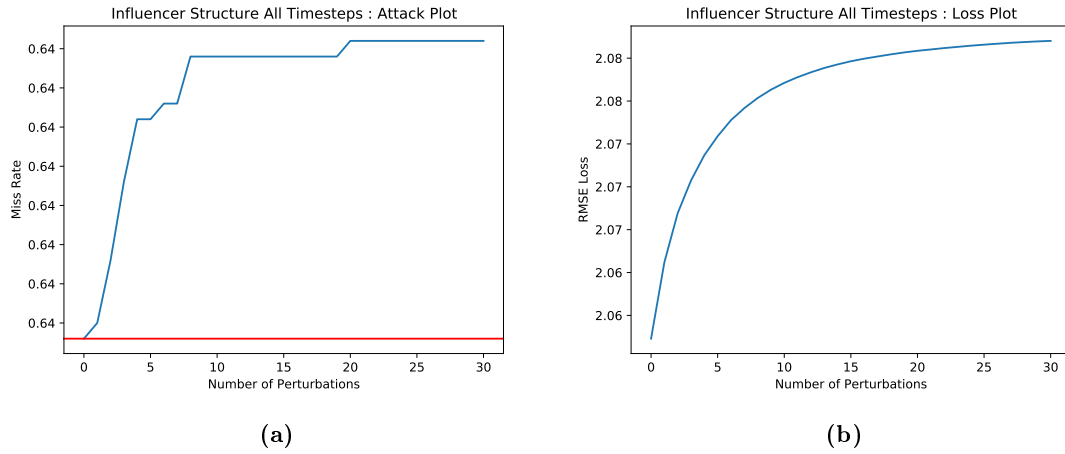
Abbildung C.22: (a) Miss Rate für indirekte strukturelle Angriffe auf alle Zeitschritte auf das GCN Modell. (b) Verlauf des Fehlerterm für indirekte strukturelle Angriffe auf alle Zeitschritte auf das GCN Modell
