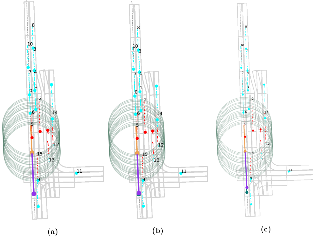
Abbildung 5.21: (a) GCN: \Delta FDE : 0.02 , (b) GAT-2: \Delta FDE : 0.60, (c) GAT-4: \Delta FDE : 3.31
