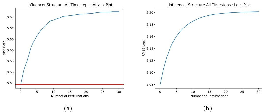
Abbildung C.23: (a) Miss Rate für indirekte strukturelle Angriffe auf alle Zeitschritte auf das GAT-2 Modell. (b) Verlauf des Fehlerterm für indirekte strukturelle Angriffe auf alle Zeitschritte auf das GAT-2 Modell
