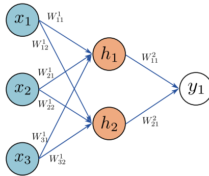
Abbildung 2.10: Unverändertes feedforward neuronales Netz: Die Eingabe fester Größe wird ohne Rückkoppelungen zur Ausgabe y_1 transformiert. Inspiriert durch [30].
