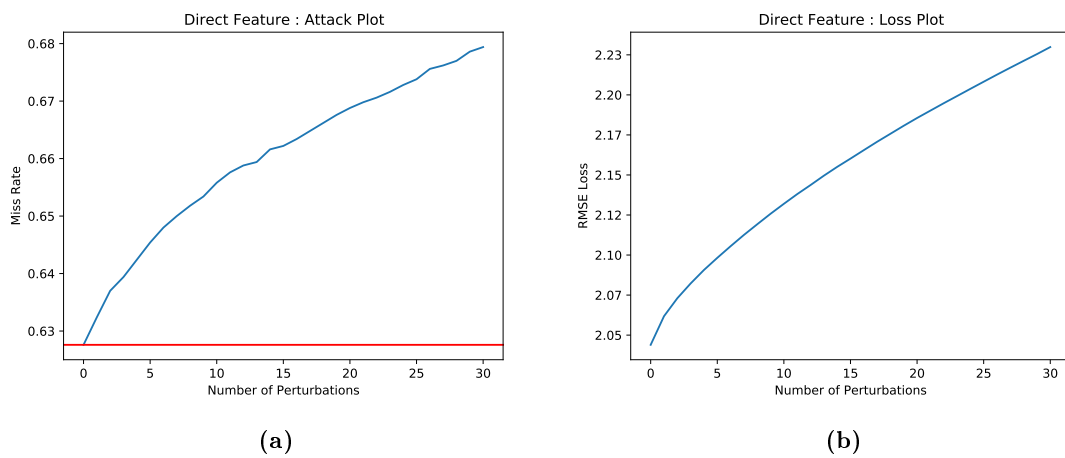
Abbildung C.9: (a) Miss Rate für direkte Featureangriffe auf das GAT-4 Modell. (b) Verlauf des Fehlerterm für direkte Featureangriffe auf das GAT-4 Modell
