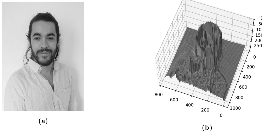
Abbildung 2.7: (a) Ein Bild nur mit Grauwerten zwischen 0 – 255 dargestellt. Je heller der Pixel, desto höher der Grauwert. (b) Dasselbe Bild dargestellt als Höhenkarte. Die Z-Koordinate kodiert die Grauwerte.
