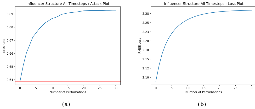
Abbildung C.24: (a) Miss Rate für indirekte strukturelle Angriffe auf alle Zeitschritte auf das GAT-4 Modell. (b) Verlauf des Fehlerterm für indirekte strukturelle Angriffe auf alle Zeitschritte auf das GAT-4 Modell
