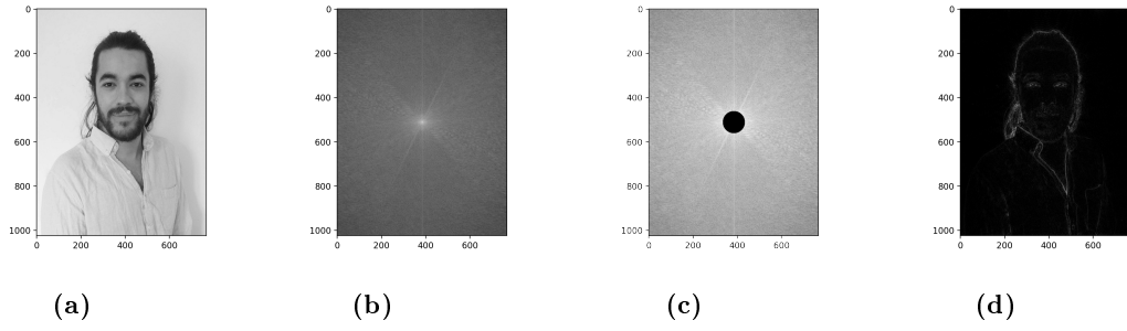
Abbildung 2.8: Filterung eines Signals im Frequenzspektrum: (a) Ein Grauwert Bild. (b) Das Frequenzspektrum des Bildes. Je heller der Eintrag, desto größer ist die Amplitude des Frequenzanteils. (c) Der schwarze Kreis in der Mitte symbolisiert einen Hochpassfilter. Alle kleinen Frequenzen werden ausgeschnitten . (d) Das gefilterte Bild, nach dem das Frequenzspektrum mit Hilfe der inversen Fouriertransformation zurück in die räumliche Darstellung transformiert wurde.
