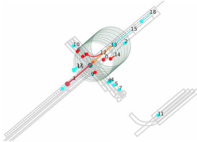
Abbildung 4.4: Visualisierung einer Vorhersage: Observationsradius (grün) des Agenten für 20 Zeitschritte. Der Radius beträgt 20 Meter. Verkehrsteilnehmer, die zum gemessenen Zeitpunkt innerhalb des Sichtradius waren, sind mit einem roten Punkt markiert. Die beobachtete Trajektorie des Agenten ist orange, die Vorhersage in grün und die wahre Bewegung rot.
